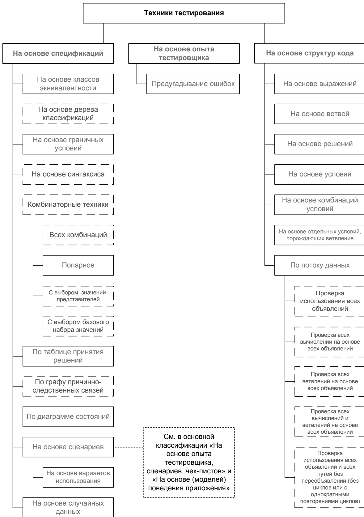
Рисунок 2.3.k — Классификация тестирования согласно ISO/IEC/IEEE 29119-4 (русскоязычный вариант)
