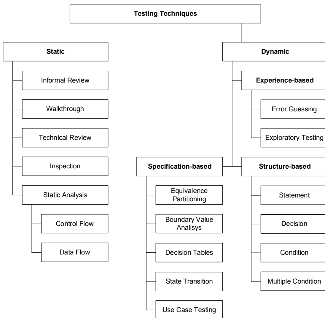
Рисунок 2.3.j — Классификация тестирования согласно книге « Foundations of Software Testing: ISTQB Certification » (Erik Van Veenendaal, Isabel Evans) (англоязычный вариант)
