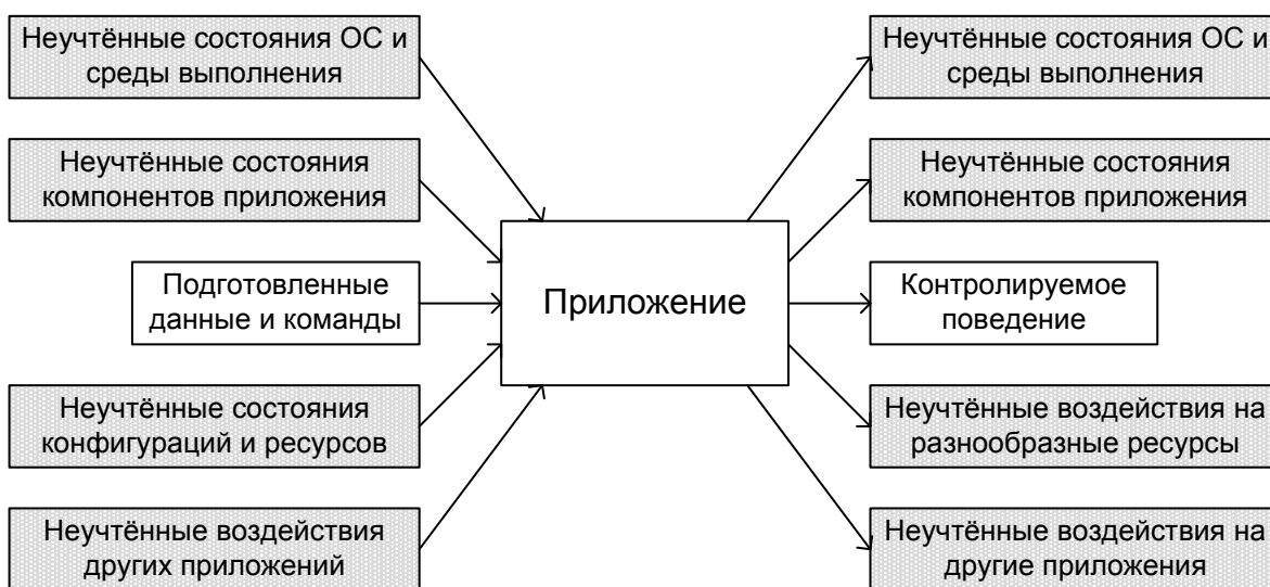
Рисунок 2.7.h — Факторы, которые могут быть пропущены тестированием на основе тест-кейсов 363
