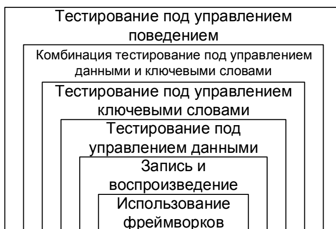
Рисунок 3.2.b — Иерархия технологий автоматизации тестирования
