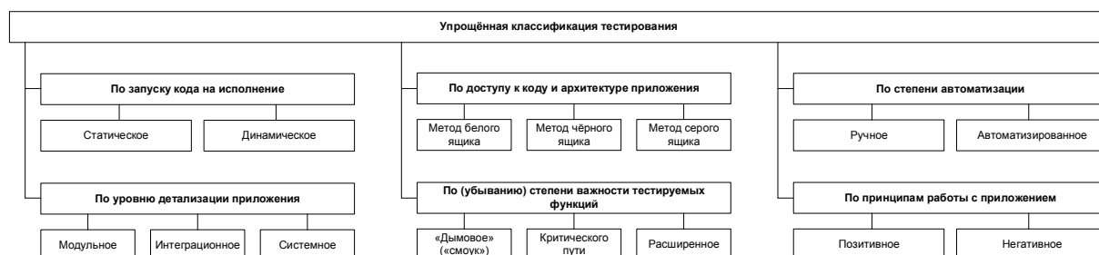
Рисунок 2.3.a — Упрощённая классификация тестирования
