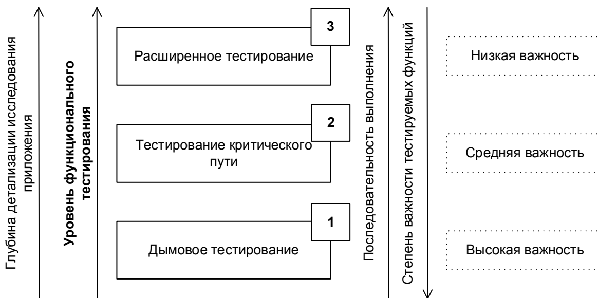
Рисунок 2.3.h — Классификация тестирования по (убыванию) степени важности тестируемых функций (по уровню функционального тестирования)
