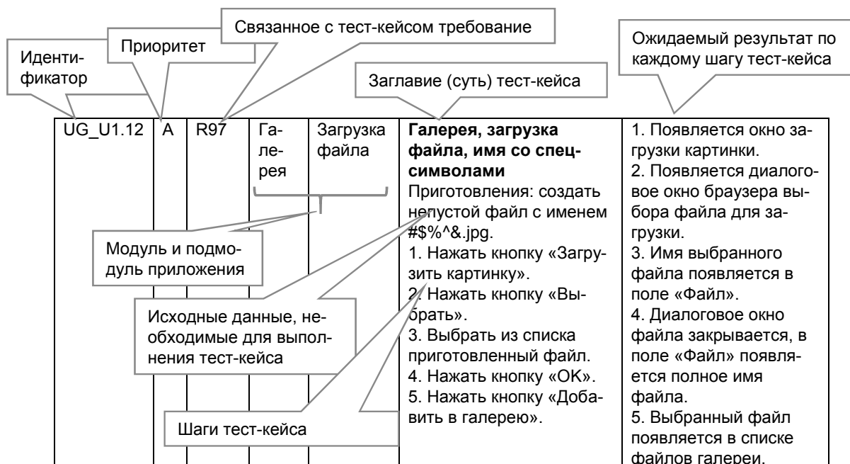
Рисунок 2.4.б — Общий вид тест-кейса
