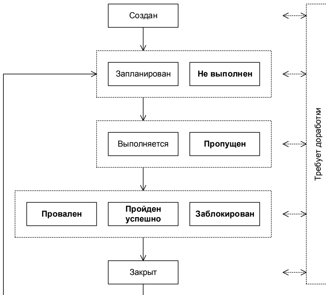
Рисунок 2.4.a — Жизненный цикл (набор состояний) тест-кейса
