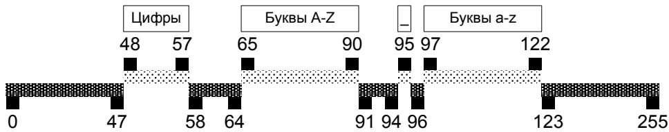
Рисунок 2.7.c — Неудачный способ поиска классов эквивалентности для наборов допустимых и недопустимых символов (коды символов приведены по ASCII-таблице)
